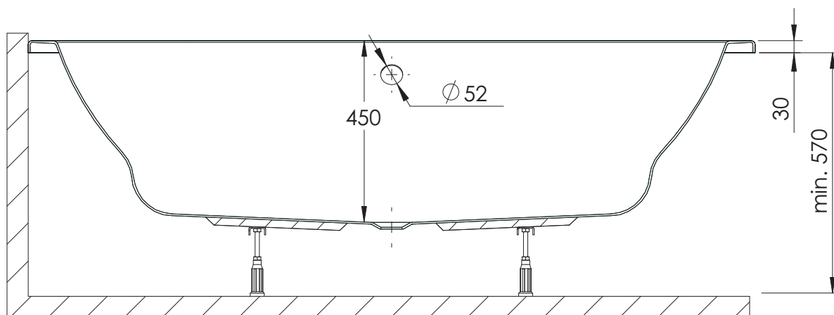
ŘEZ A-A
